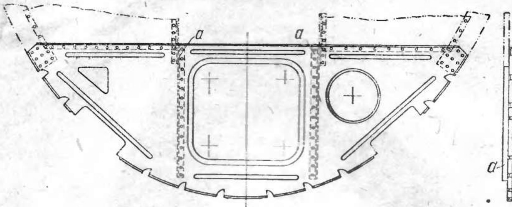
Фиг. 148. Деталь № 1 шпангоута фюзеляжа (пунктиром нанесены соседние детали шпангоута). а—приклепанные к спинке детали прессованные угольники.
