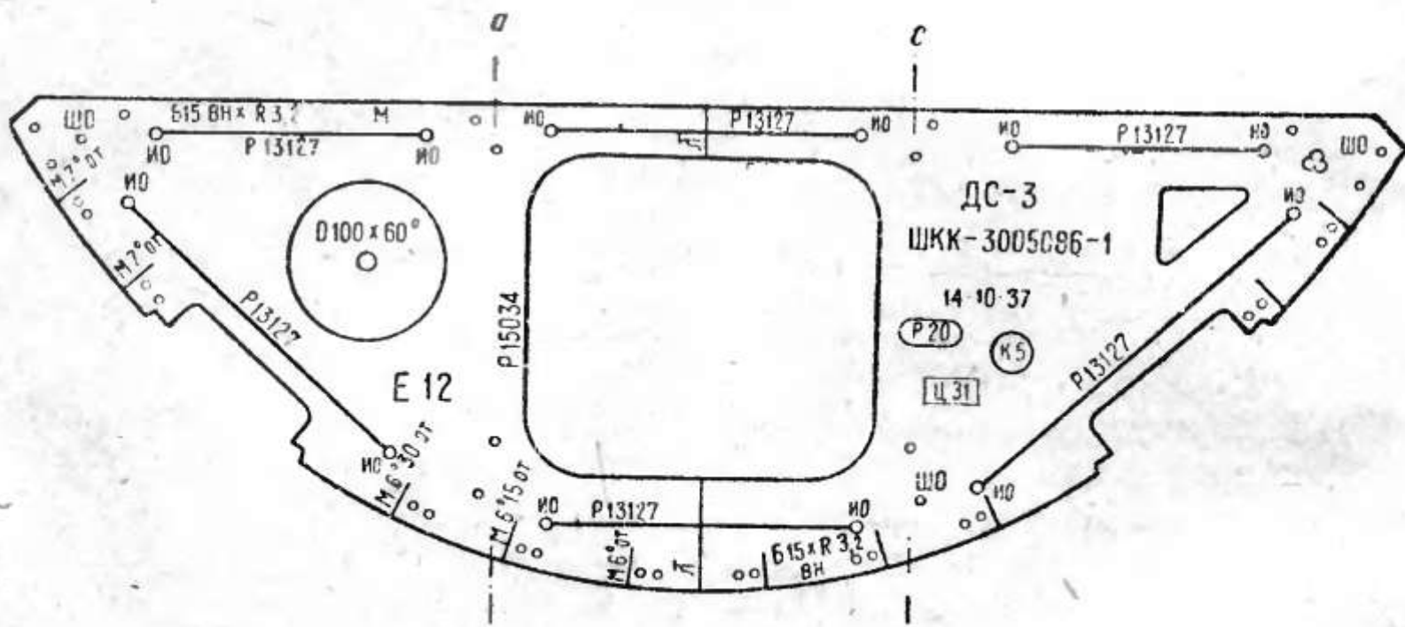
Фиг. 148. Деталь № 1 шпангоута фюзеляжа (пунктиром нанесены соседние детали шпангоута). а—приклепанные к спинке детали прессованные угольники.
